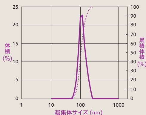
水中に分散したAEROXIDE®の粒径分布
