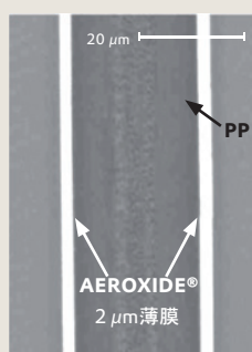
AEROXIDE®でコーティングしたセパレーターの断面SEM画像
